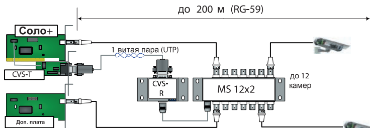
Рис. 2. Удаленное размещение MS 12x2 до 200 м.
