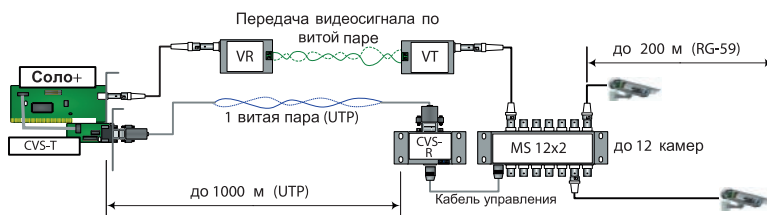
Рис. 5. Удаленное размещение MS 12x2 до 1000 м.
