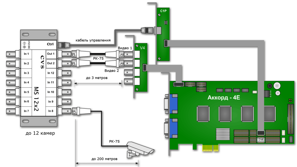
Рисунок 1. Схема подключения оборудования.
